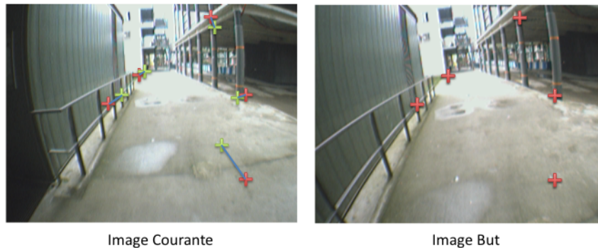
Figure 5.4: Illustration du principe de l'asservissement visuel: l'erreur entre une image courante et une image but (écart entre les croix rouges et vertes ici) est utilisée pour calculer une commande qui permettra au robot d'atteindre la position correspondant à l'image but.
