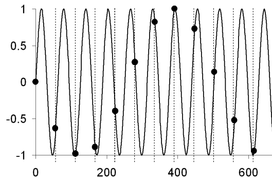
FIGURE 1.5 – Phénomène d'aliasing sur un signal 1d
