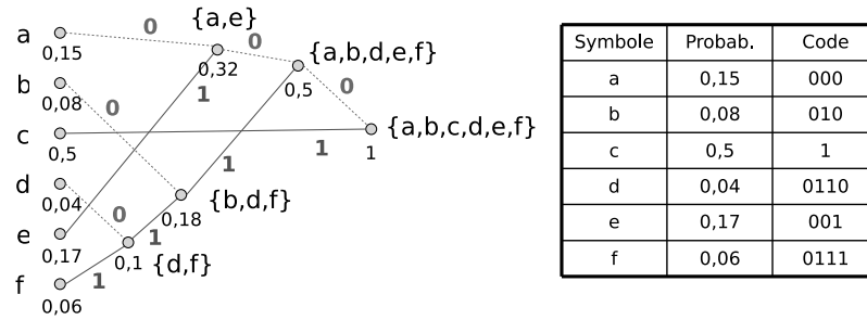
FIGURE 1.12 – Algorithme de codage de Huffman. A gauche : arbre binaire construit par l’algorithme d’encodage. A droite : tableau montrant pour chaque symbole (valeur) s , sa probabilité empirique dans I ( P_I(s) ), et le code de Huffman résultant.
