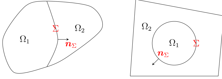
FIGURE 1.1 – Exemples de partition d'un domaine de \mathbb{R}^2
