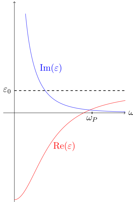
FIGURE 6.1 – Parties réelles et imaginaires de la permittivité d'un métal en fonction de la fréquence
