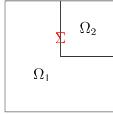
FIGURE 8.5 – Domaine symétrique : contraste \kappa_\sigma = -1.001 .
